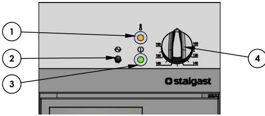
Rysunek 8 Elementy sterujące urządzeniem
