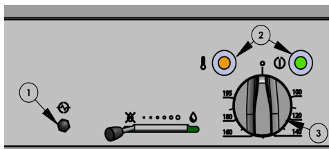
Rys. 10. Elementy sterujące urządzeniem
